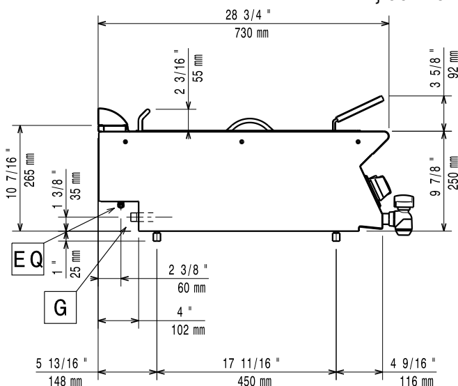
Zij aanzicht
